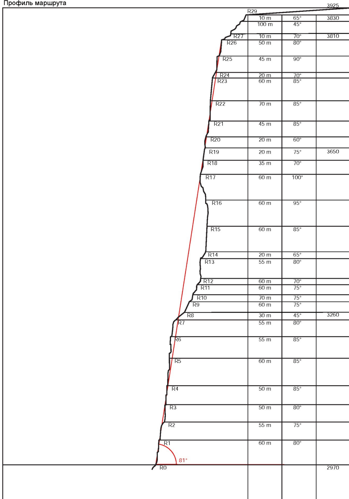
Профиль маршрута
